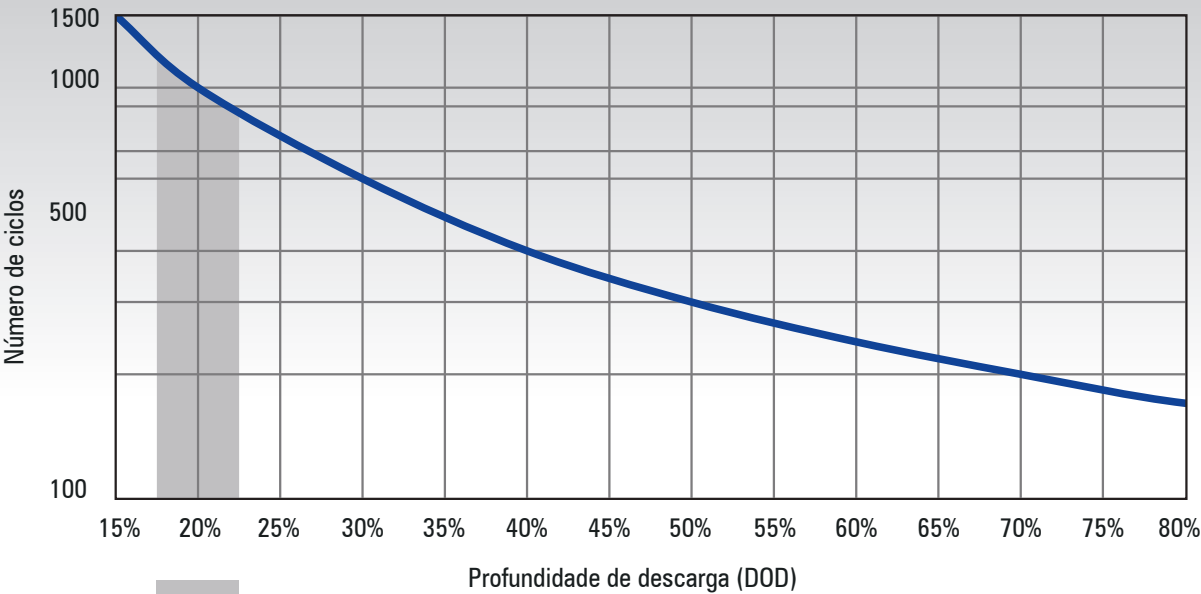
Número de ciclos em função da profundidade de descarga
