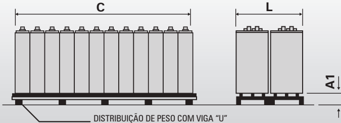
DUAS FILAS EM NÍVEL (BATERIAS 2750 a 3000 Ah)
